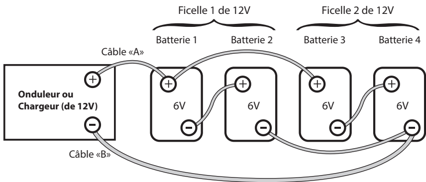
Figure 7.4 : Connexion série-parallèle
