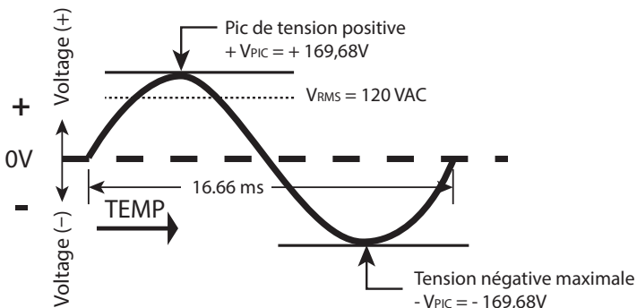
La Fig. 5.1: Une Forme d'Onde Sinusoïdale Pure de 120 VCA, 60 Hz
