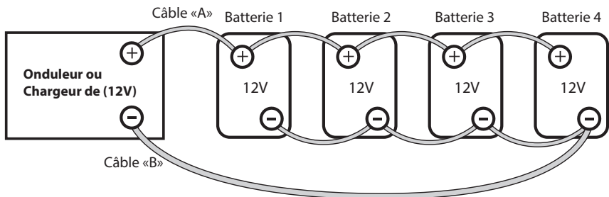
Figure 7.3: Connexion parallèle
